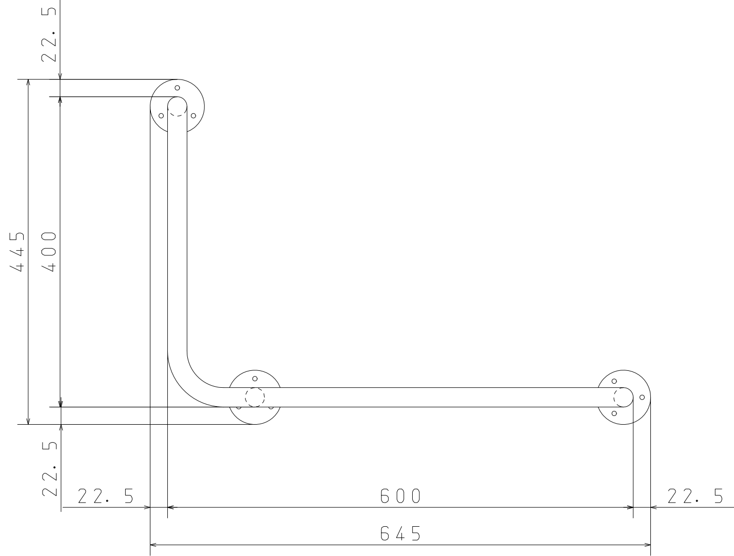
正面図
